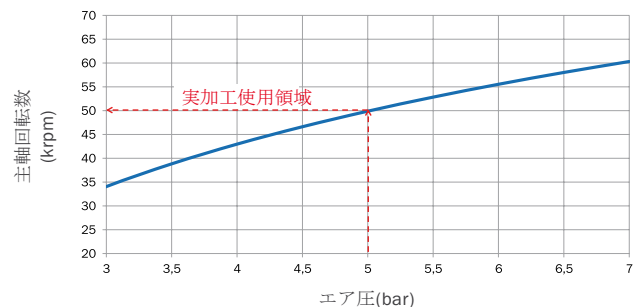
主軸回転数/エア圧
