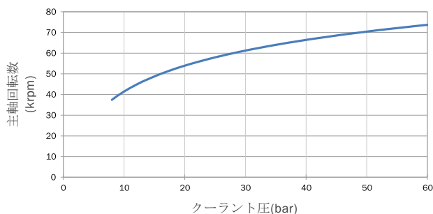
主軸回転数/クーラント圧
