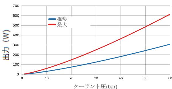
出力/クーラント圧
