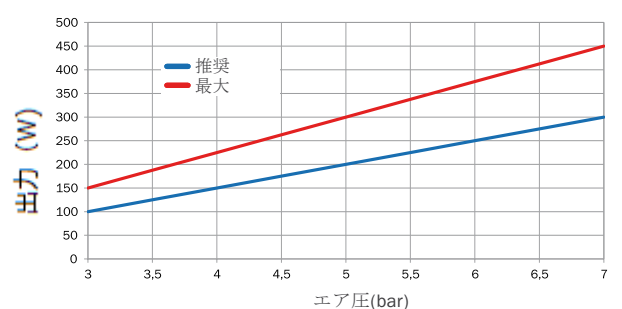
出力/エア圧
